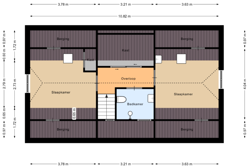
1e Verdieping
